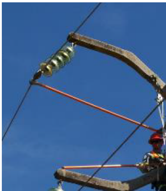
Figura 3 - Afastamento da fase B em estrutura triangular.
