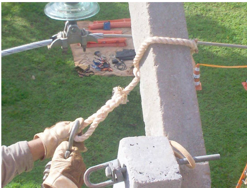
Figura 2 – Instalação da corda de serviço e a carretilha acima do local onde serão executados os serviços.
